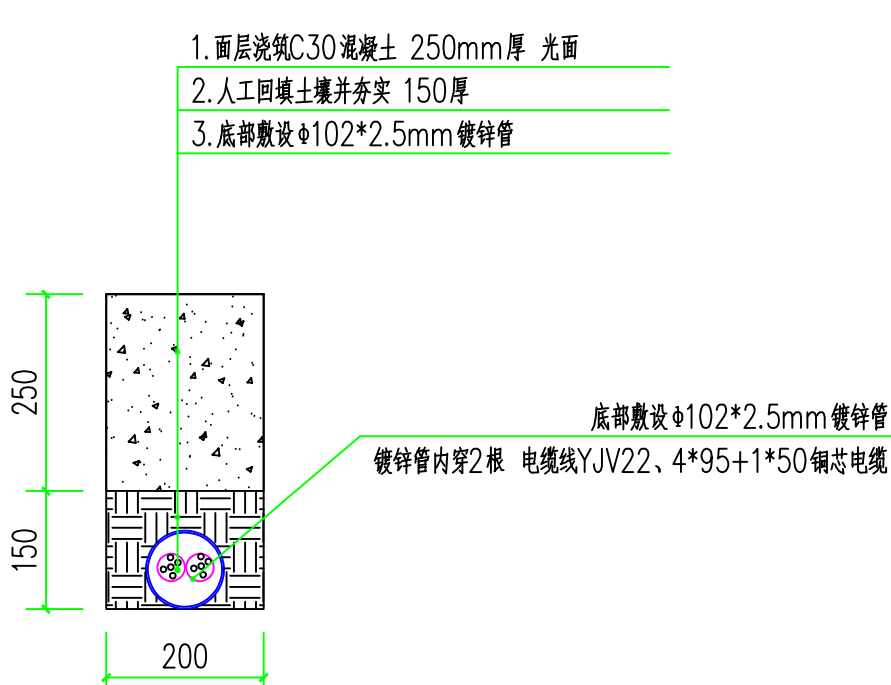
1-1电缆沟做法示意图
