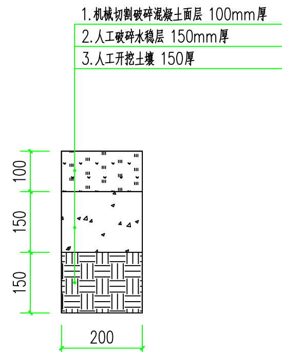
1-1电缆沟开挖示意图
